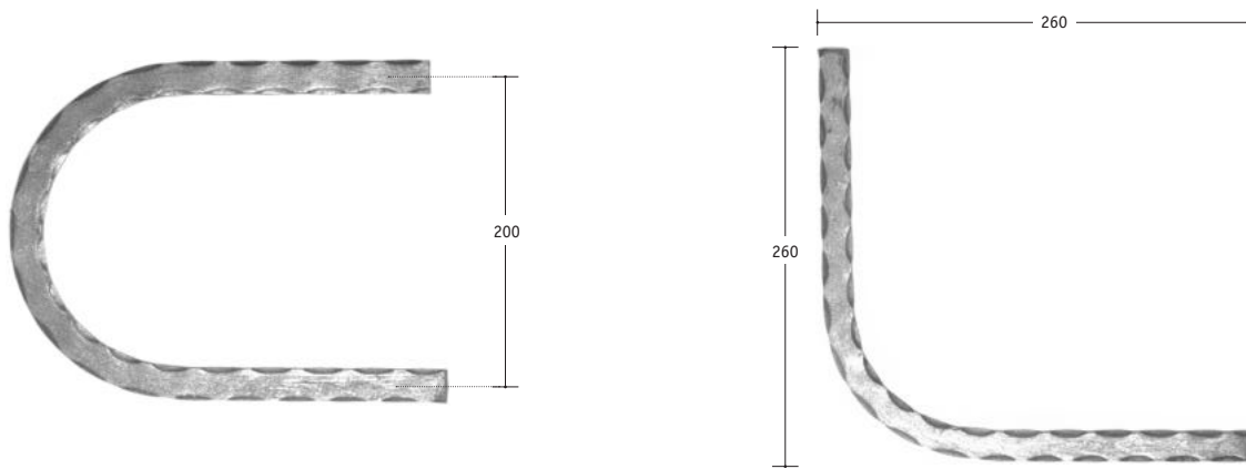
Krümmling, 180°, einseitig gehämmert
