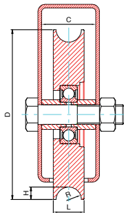
Laufrolle U-Profil , Laufrolle mit Kugellager, Form U, Bolzen M14 x 70
