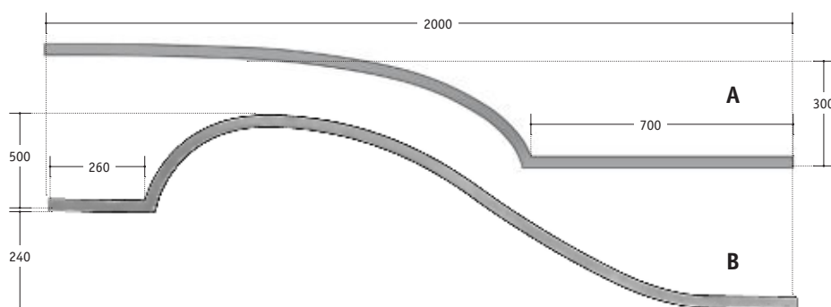
Rohrbogen
