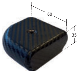
Pfostenabschluss, mit Gewinde M10
