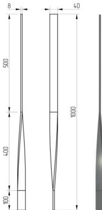
Geländerstab »Akzent-2« , aus Flacheisen 40 x 10 mm, Länge: 1000 mm, glatt, asymmetrisch, nicht mittig, 90° gedreht
