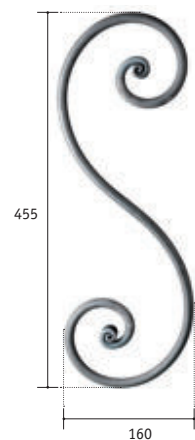
S-Bogen, glatt, Enden gleich eingerollt
