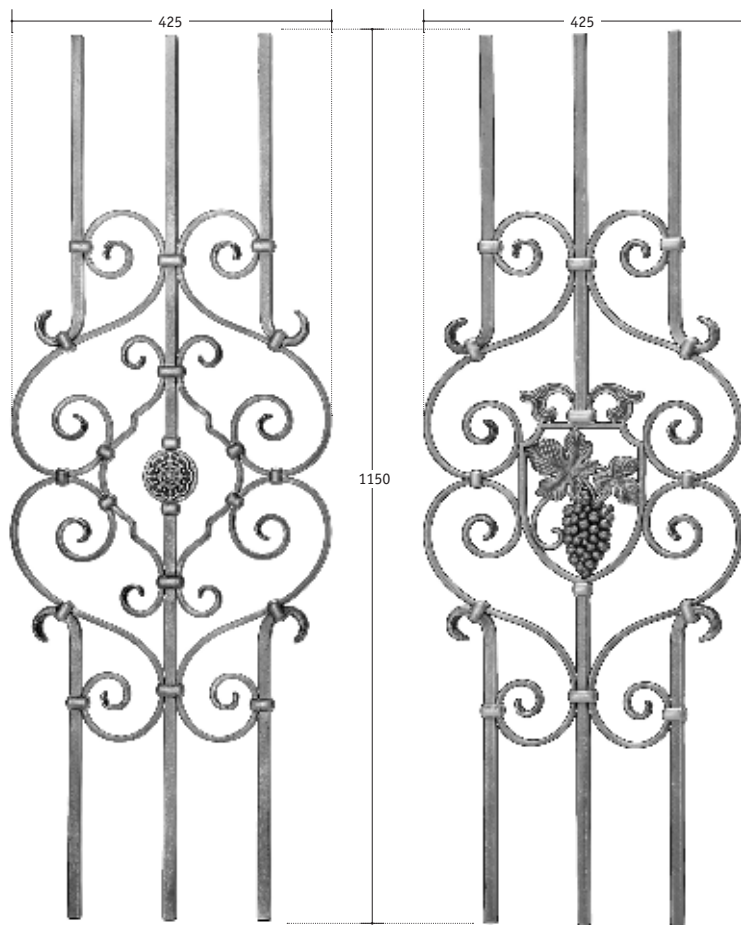
Zierelement mit Blumenornament
