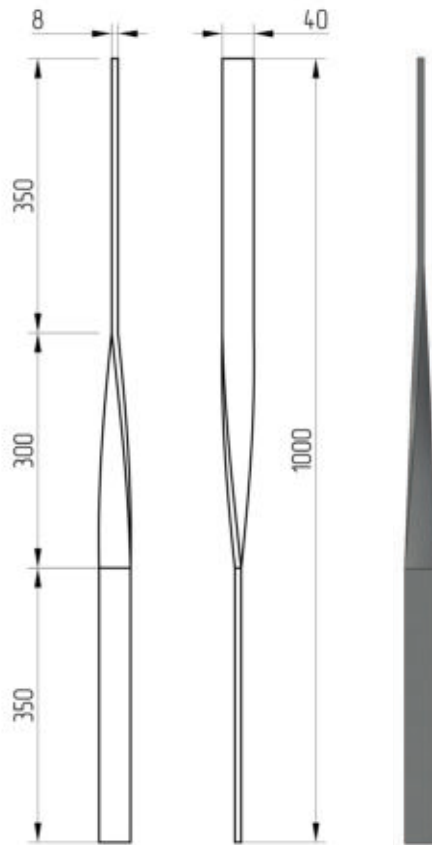
Geländerstab »Akzent-1« , aus Flacheisen 40 x 10 mm, Länge: 1000 mm, glatt, mittig 90° gedreht
