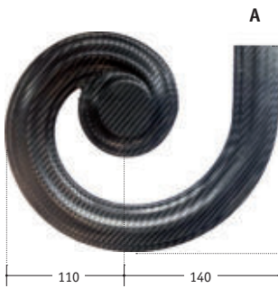
Handlauf-Anfangsstück
