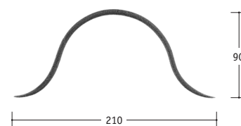
Ziermantel, glatt
