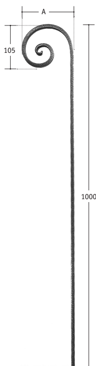
Schneckenstab, glatt
