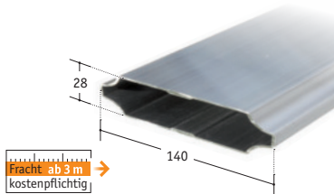
Alu-Verkleidungsprofile, 140 x 28 mm Länge: 6000 mm
