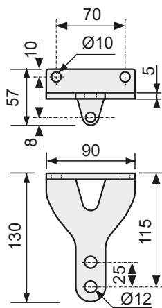
Montageteil motorseitig
