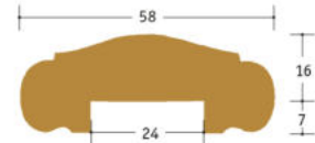
Profil-Handlauf - Typ 3
