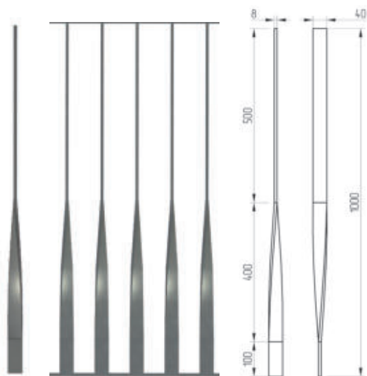
Design- stäbe AKZENT
