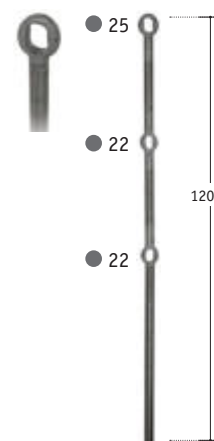
Lochstab, 3 x Oval-Lochung für 1 x 25 mm & 2 x 25 mm, für Treppen
