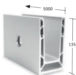
TURBOFLEX Ganzglasgeländersystem (1,0 kN) Glasprofil Modell TF-6621 für Seitenmontage
