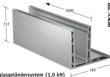
TURBOFLEX Ganzglasgeländersystem (1,0 kN) Glasprofil Modell TF-3620, für Bodenmontage
