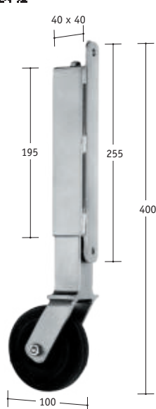
Torlaufrolle, leicht, feuerverzinkt, mit Teleskop-Federbein, max. Rollenbelastung: 70 kg, Fe- derweg 60 mm, Federkraft: 55 kg, Rolle mit Vorspannung montieren!
