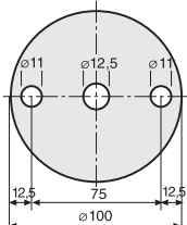
Ronde, Stahl roh, mit 3 Bohrungen
