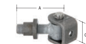
Torband mit kurzem Gewinde, Einschweißmutter und geschlosse- nem Bügel, Schraube feuerverzinkt, Bolzen V2A
