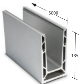
TURBOFLEX Ganzglasgeländersystem (1,0 kN) Glasprofil Modell TF-6620, für Bodenmontage
