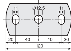
Ankerplatte, Stahl roh, oval, mit 3 Lochungen
