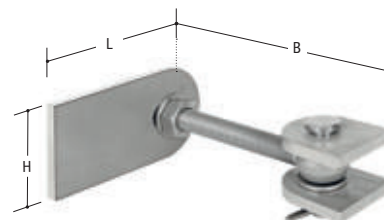
Torband V2A, 180° verstellbar, inkl. Schrauben und Muttern
